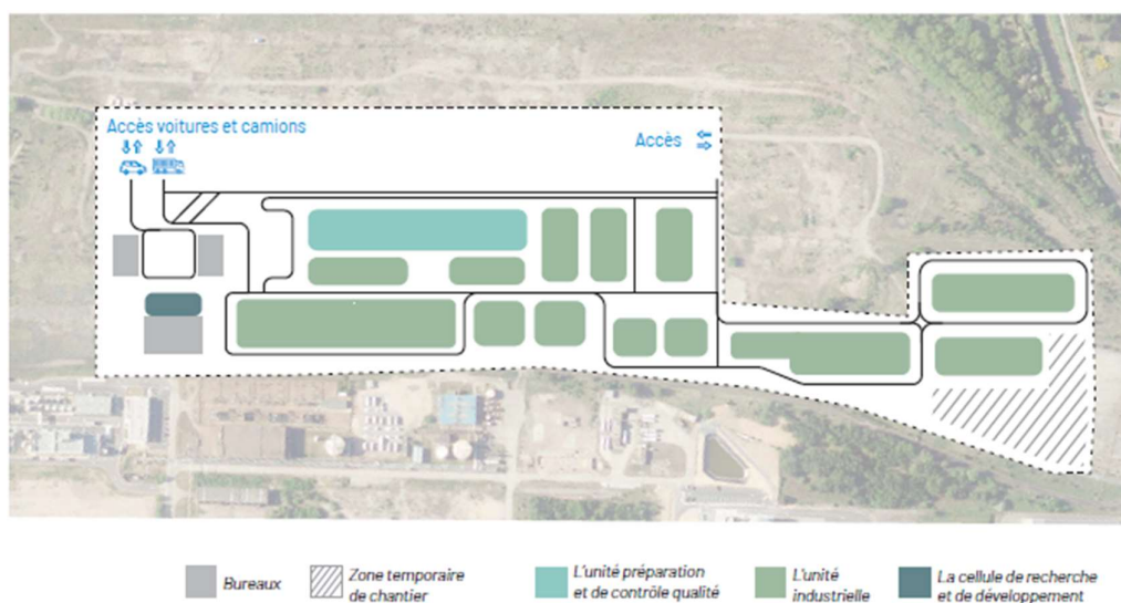
Schéma d'implantation du projet (source : dossier du Maitre d'Ouvrage)
